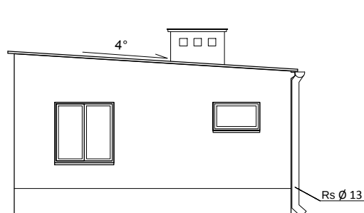
ELEWACJA WSCHODNIA
